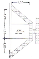
DETALHE - 02 RAMPA
